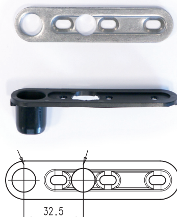
Mocowanie i utrzymywanie zestawu w pozycji nocnej wentylacji.
