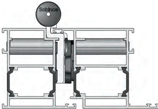
Avec ancrages à clamer
