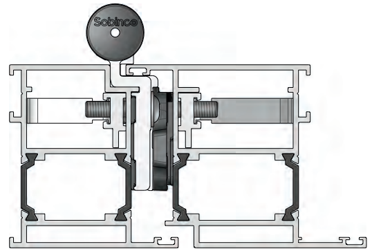
Avec pièce de serrage
